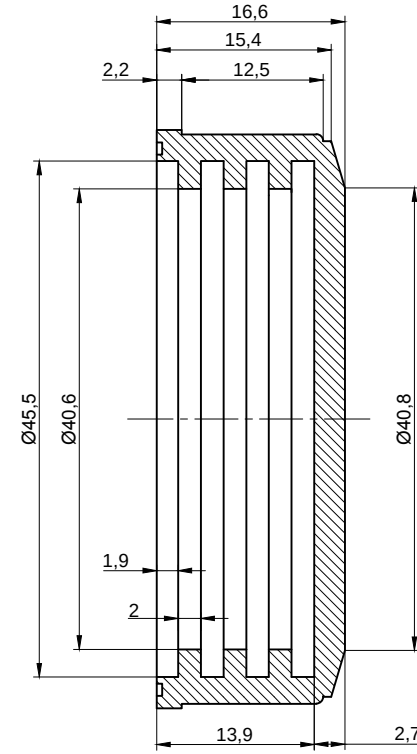
A-A KESİTİ
