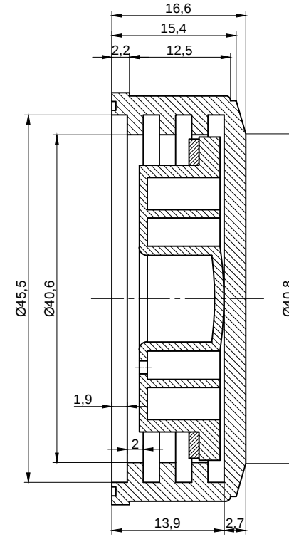
A-A KESİTİ
