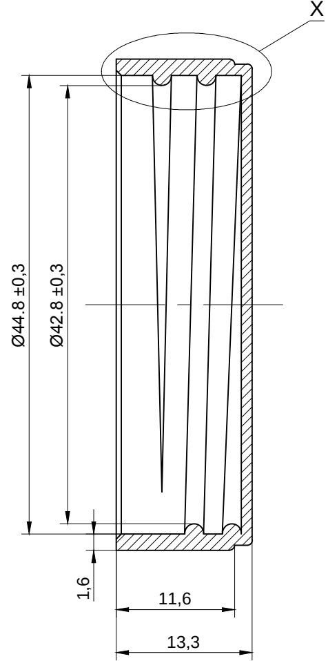
A-A KESİTİ
