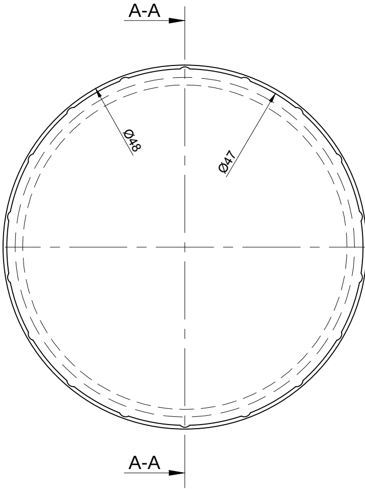
X DETAYI
