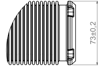
DETAY A ÖLÇEK 2 : 5
